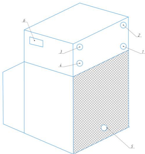
Рис. 3 Панель управления для моделей MQ20,40,60,90,120
